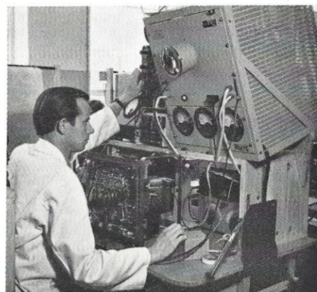
Kontrol af modtagerens „hjerter“ „Tidsbasismålepladsen“.
