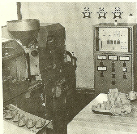
Den nye sprøjttestøbemaskine hos legetøjsfabrikken Bambola i Tåstrup er elektronstyret. Automatikken er baseret på Philips Norbit-systemer og er sammenbygget i skabet til højre.
