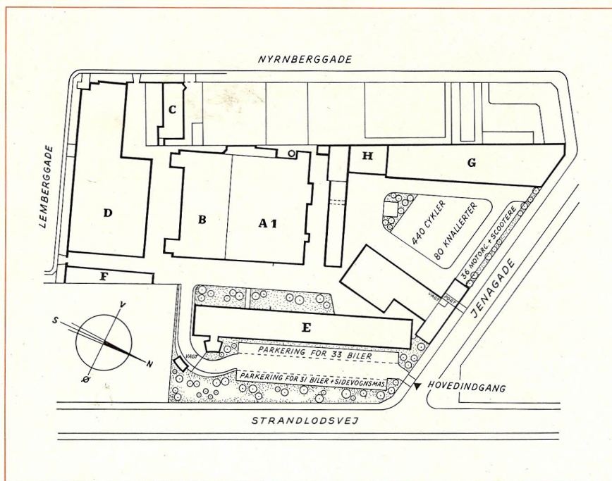
Her er en grundplan af hele fabriksarealet, som det vil tage sig ud, når det nuværende byggeri er afsluttet.
