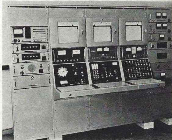
Noget af det mest interessante på el- og atomudstillingen: et Philips-panel til betjening af en atom-reaktor. Panelet er ca. 2\frac{1}{2} m langt.
