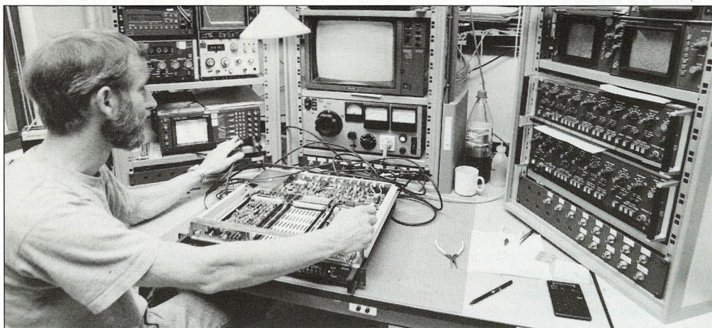
Erling Johansen fra Transmission Team er i gang med sluttet af en PM 5638. For dem der har forstand på den slags: Det er et apparat, som laver et RGB-signal om til et composite video signal.
