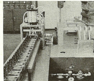
Emnerne føres automatisk ind i punktvejseren, hvor de bliver svejset på 4 steder samtidigt. Tidligere måtte man svejse eet punkt ad gangen manuelt.
